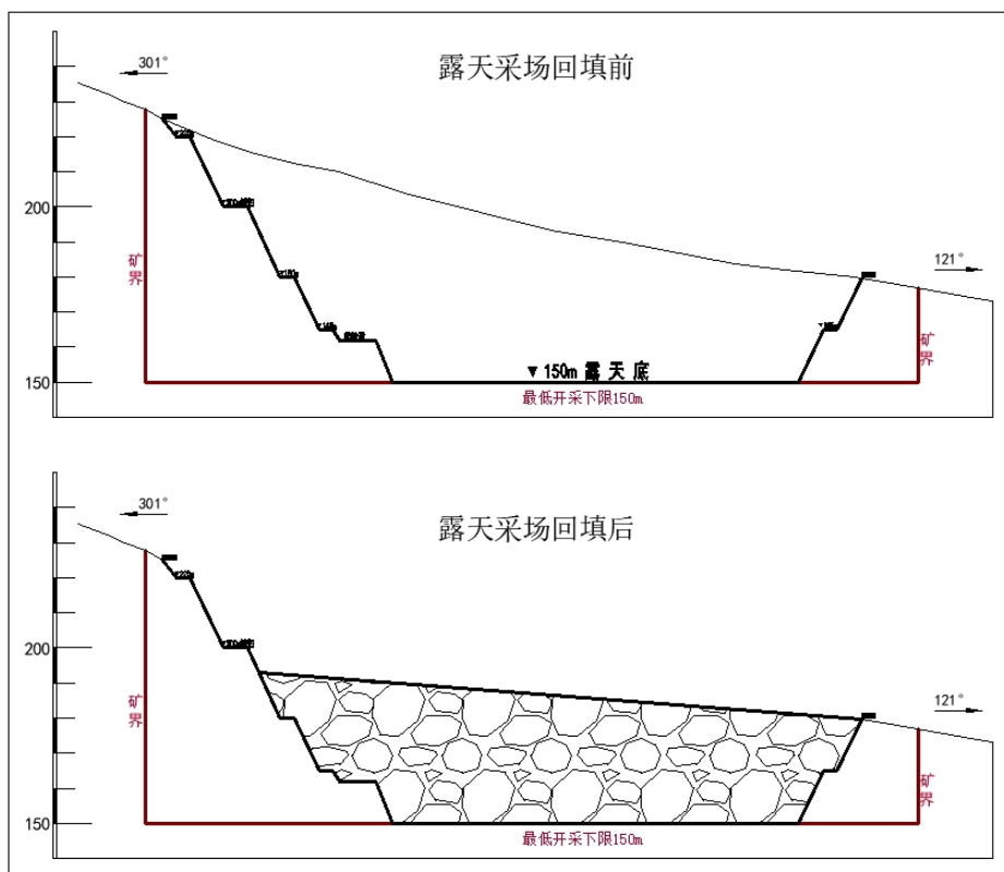
图 5-1 露天采场回填示意图
