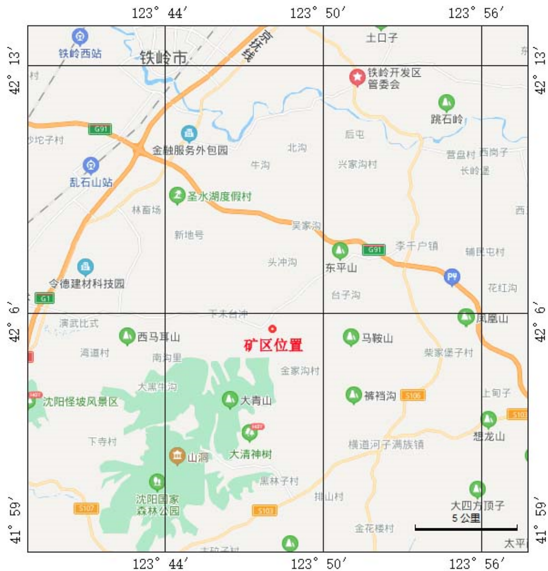
图1 矿山交通位置图
