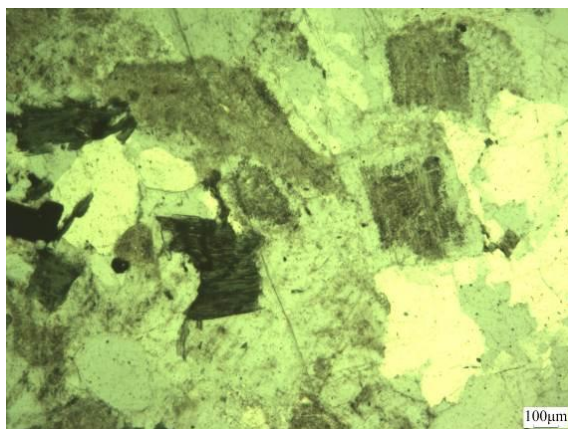
图 3-2 中细粒黑云母二长花岗岩
