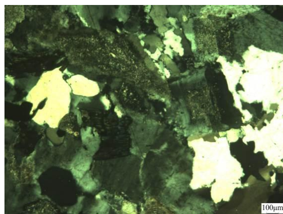
图 3-3 中细粒黑云母二长花岗岩
