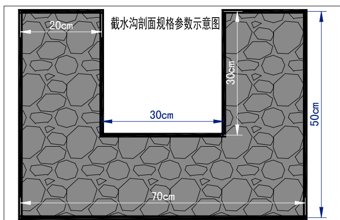
插图 5-4 截水沟剖面示意图
