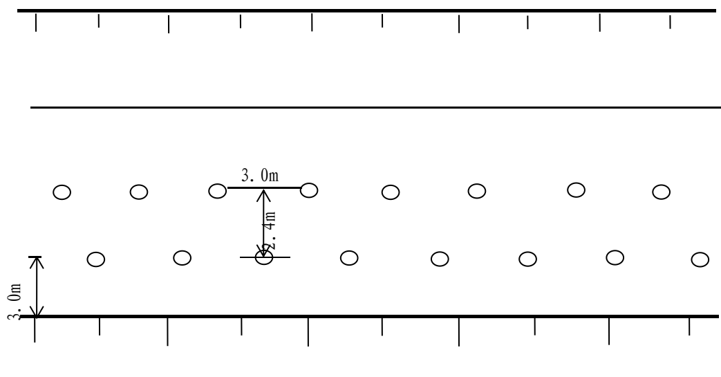
插图 5-1 爆破剖面示意图
