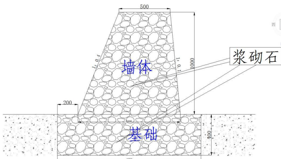
插图 5-3 浆砌挡渣墙断面示意图
