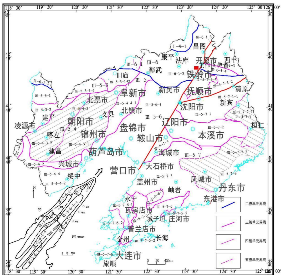
图 3-1 辽宁省地质构造单元区划图(《中国区域地质志》辽宁志, 2014)
